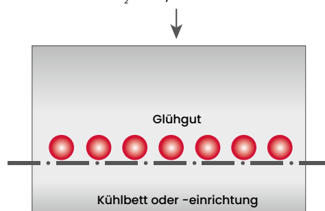
Strahlungskühlung ohne/mit Abschreckkühlung mittels Luft, \text{H}_2\text{O} , Luft + \text{H}_2\text{O} oder \text{H}_2\text{O} -Polymer-Emulsion
